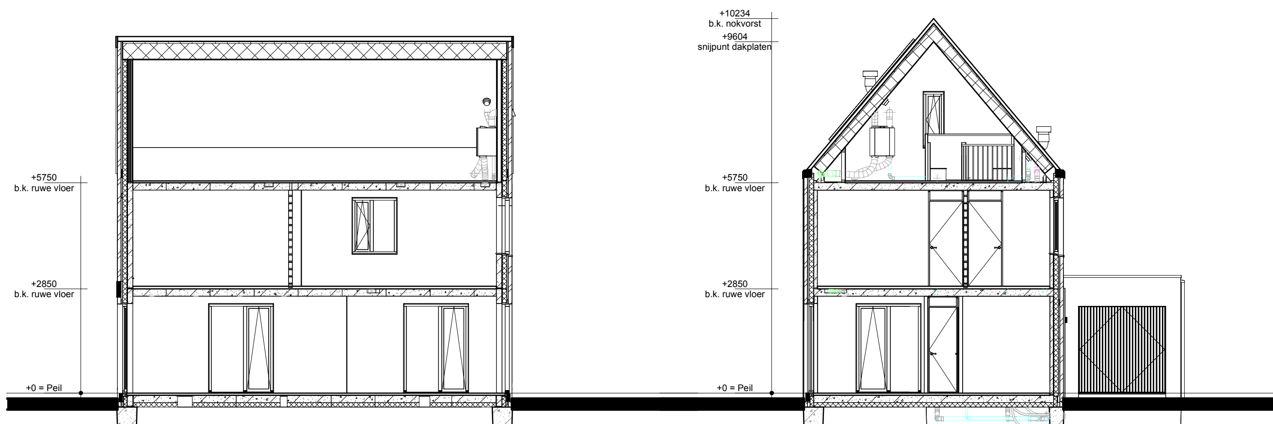
Doorsnede A1-A1
